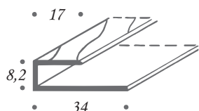
Art. PAV/TB - Terminale Quadro Profilo per porte/finestre
