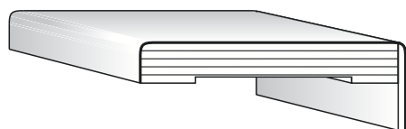
COPRIFILO c/aletta (70x10)mm - raggio 2 mm Interno utile aletta 25 mm
